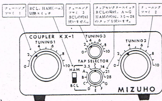
図-2 ツマミの操作方法 (図-2)
