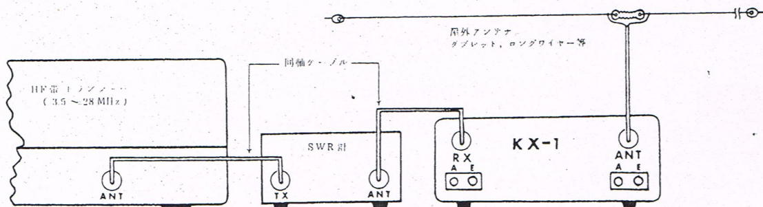
図-3 アマチュア無線局での送信機との接続方法 (図-3)
