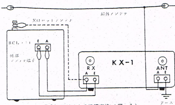
図-1 BCL ラジオとの接続方法 (図-1)
