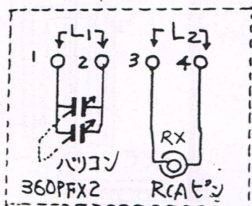
バリコンBOX
