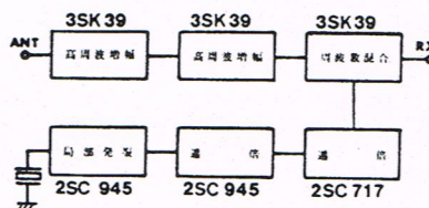
VX-1 ブロックダイアグラム
