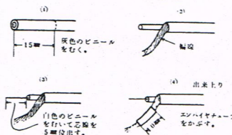
(図-1) 同軸ケーブルの処理方法
