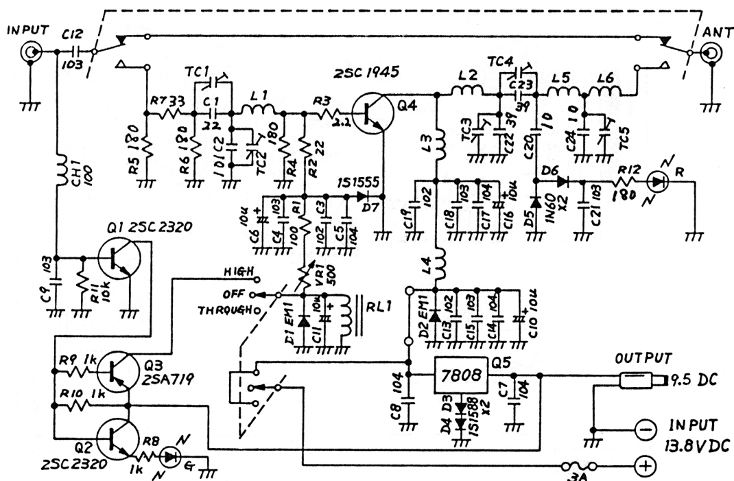
図-31 PL-28S 回路図
